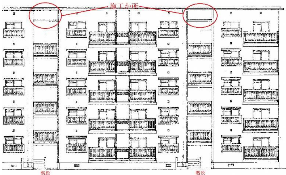
階段側立面図
